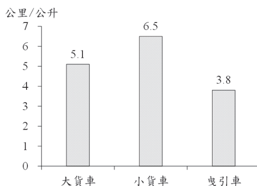
圖 1、112 年自用貨車燃油效率-按車型分
